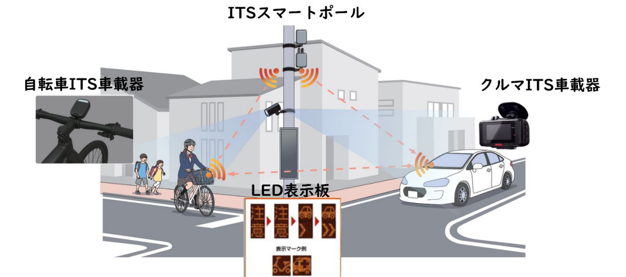
ITS スマートポールを活用した会い頭事故削減の技術
